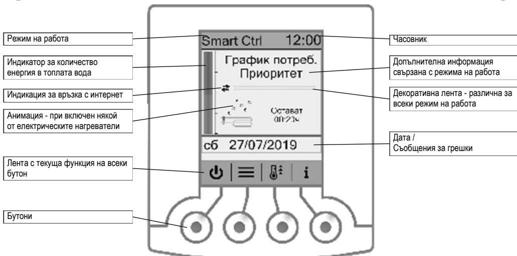
1. Вертикален монтаж
